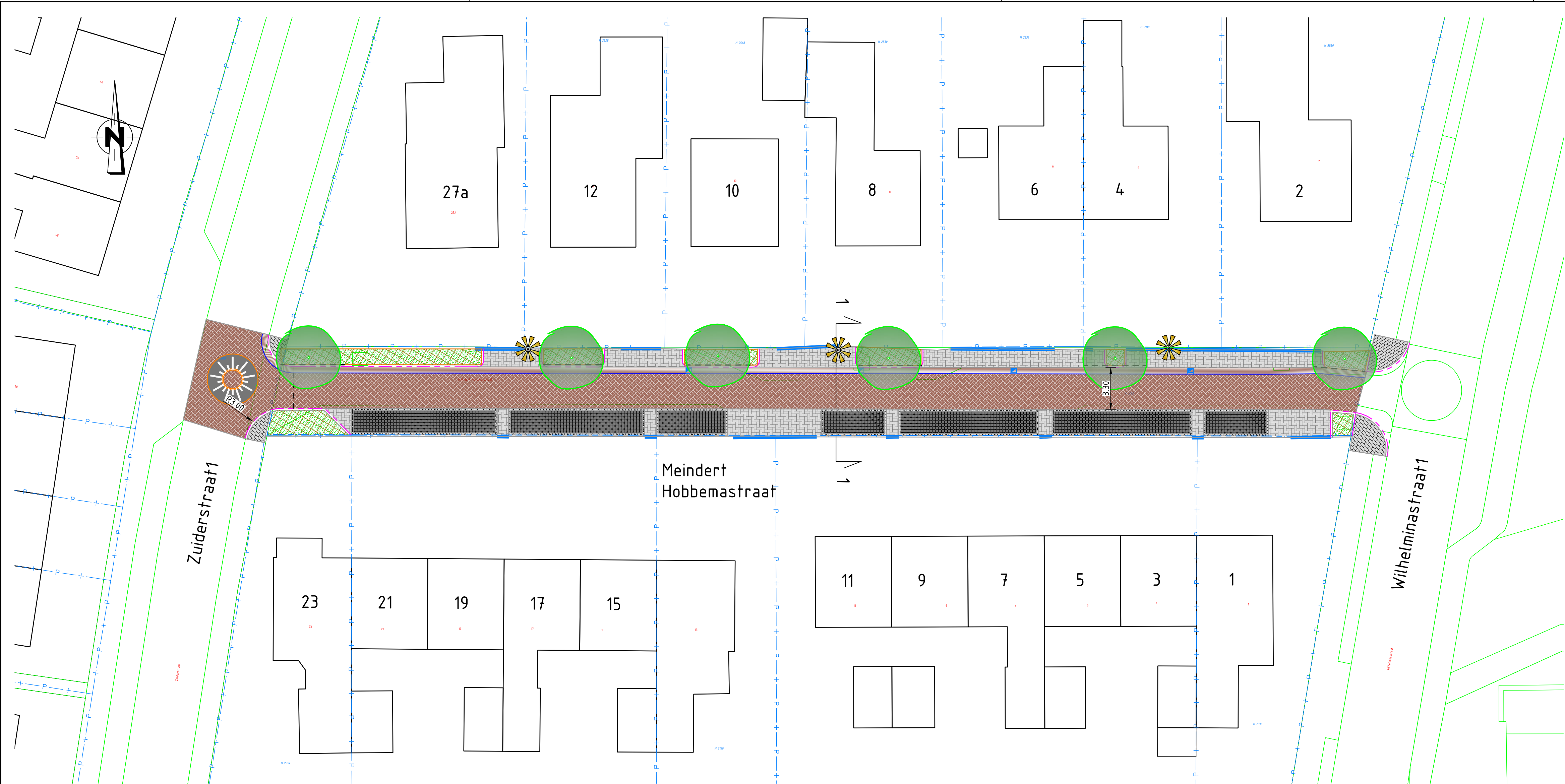
Nieuwe situatie M. Hobbemastraat (schaal 1:200)
