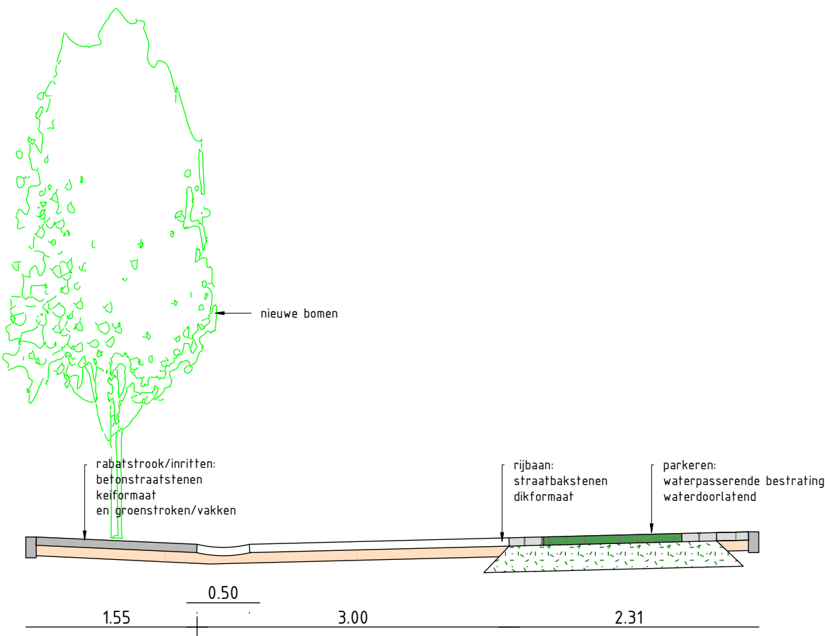
Doorsnede 1-1 (Schaal 1:50)
