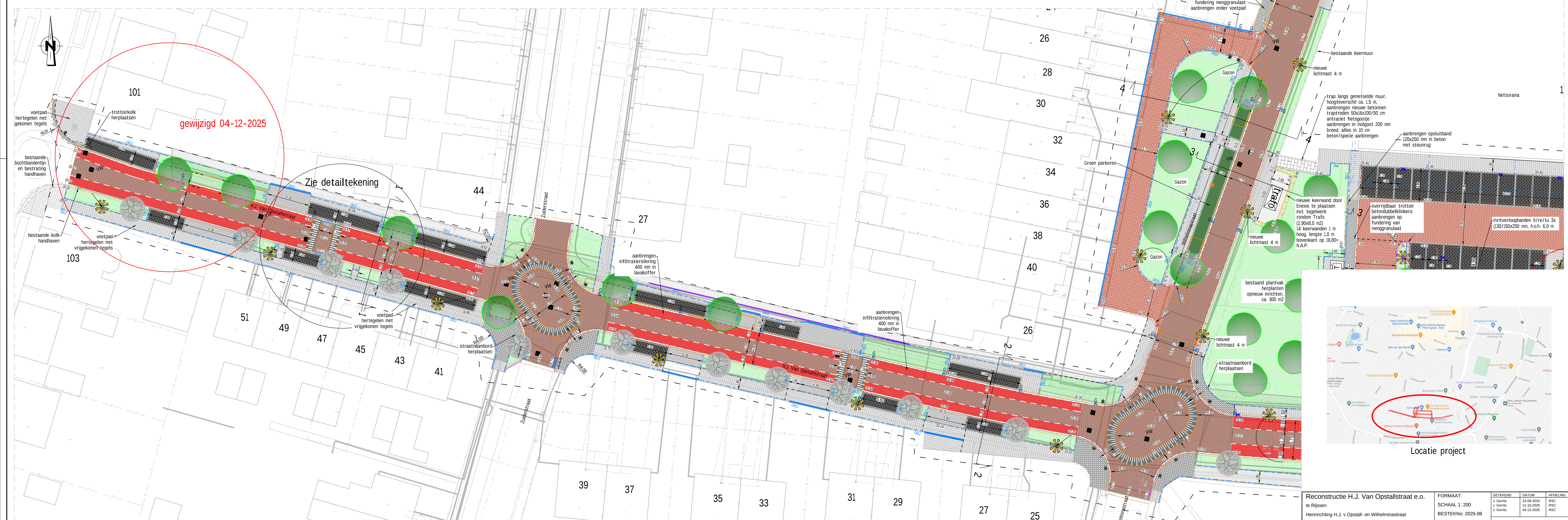
Bovenaanzicht nieuwe verhardingen en groen, deel west Esstraat -Wilhelminastraat (schaal 1:200)
